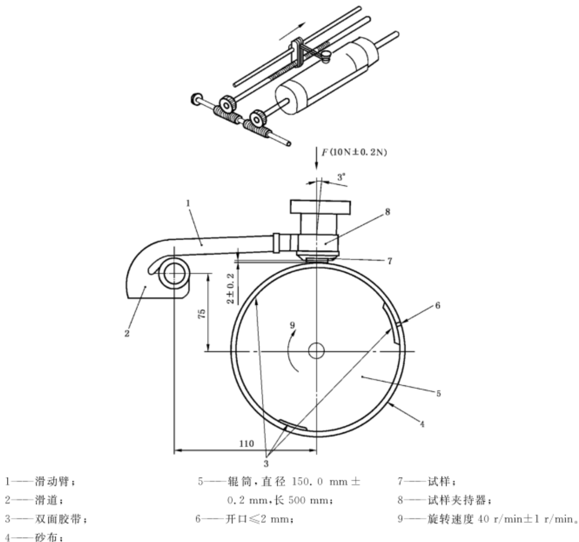
图 1 仪器结构原理图
